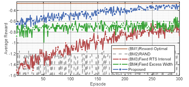
그림 2. 에피소드에 따른 제안 방안 및 비교 방안 평균 보상
